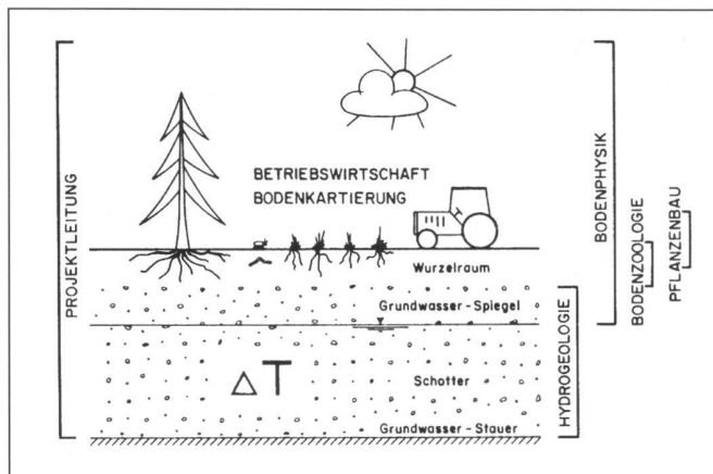
Abb. 3 und 4: Grundwassertemperatur und Pflanzenwachstum: Zusammenwirkung der verschiedenen Fachgebiete (links) und Schemaskizze des Lysimeters im Versuchsfeld Altwidn (rechts).
