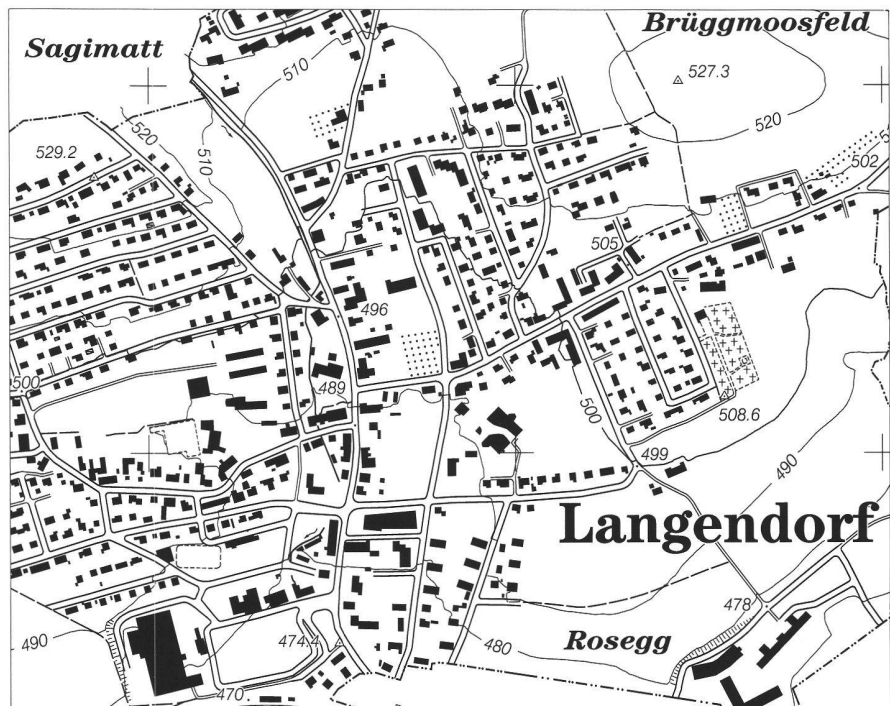
Abb. 6: Übersichtsplan 1:10000, aus dem Grunddatensatz abgeleitet, mit aufwendiger interaktiver Nachbearbeitung.
