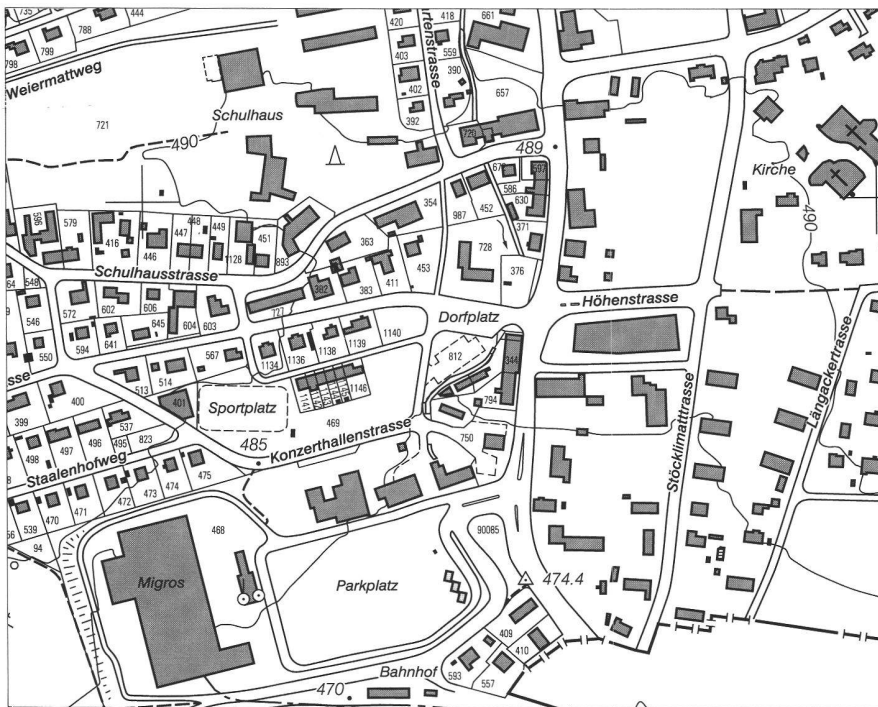
Abb. 2: Überarbeitete und generalisierte Version 1:5000.
