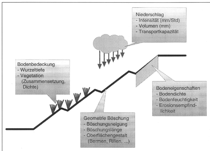
Abb. 1: Oberflächenerosion auf Hängen und Böschungen. Die vier Haupteinflussgrößen sind Niederschläge, Bodeneigenschaften, Böschungsgeometrie und -oberfläche sowie Vegetationsdecke.
