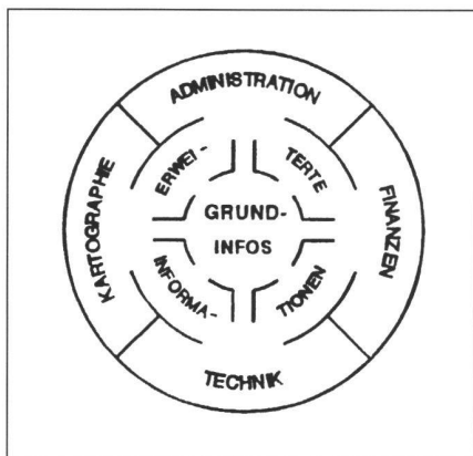
Abb. 1: GIS-Modell.
