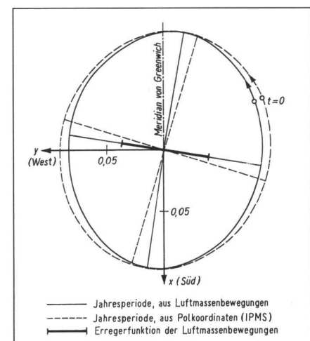
Abb. 2: Der atmosphärische Anteil der Polbewegung.
