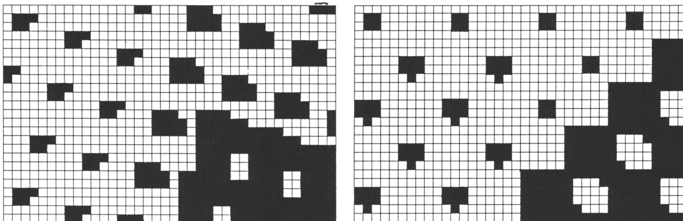
Abb. 4: Rastermuster des Cyan- und Schwarzauszuges mit 18°, resp. 45° Rasterwinkelung und einer Pixelgrösse von 25 \mu\text{m} .
