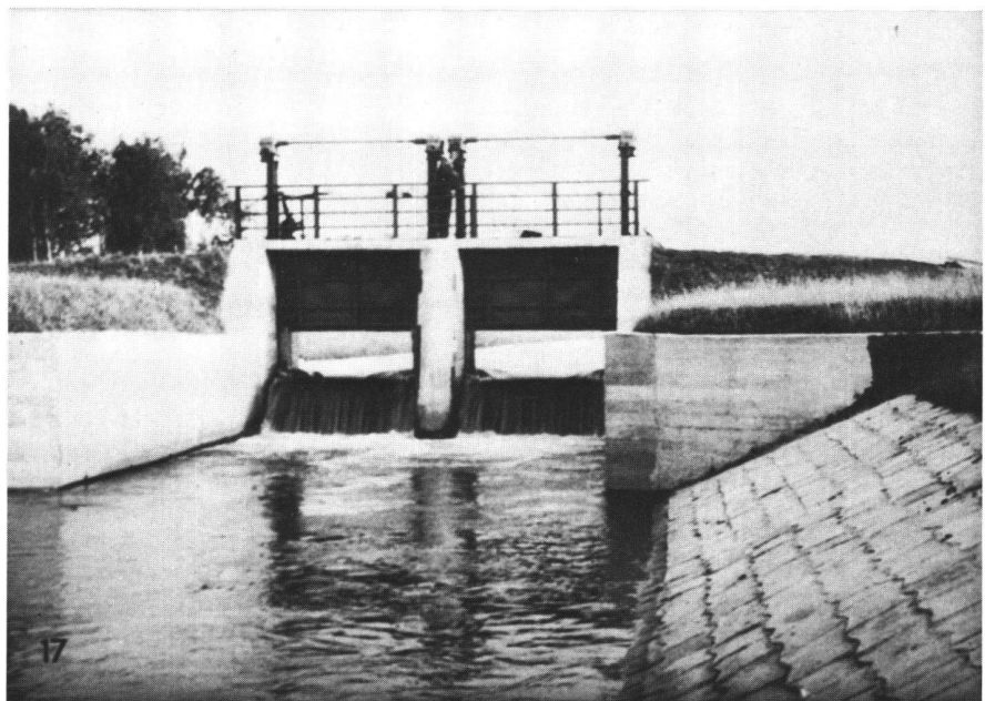
Abb. 7: Wehr im Kanal Wieprz-Krzna (Ostpolen)
