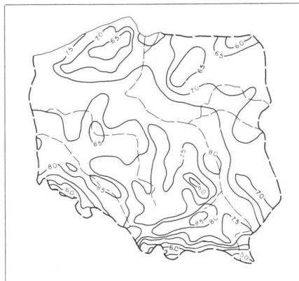
Abb. 2: Jahresisothermen auf der effektiven Höhenlage
