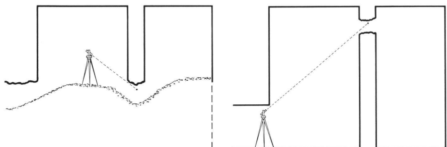
Abb. 1: Zwei Fälle, welche – in Analogie zum bekannten Schachtproblem – für eine exakte Bauaufnahme den Einsatz eines Kreiseltheodoliten erfordern würden.
