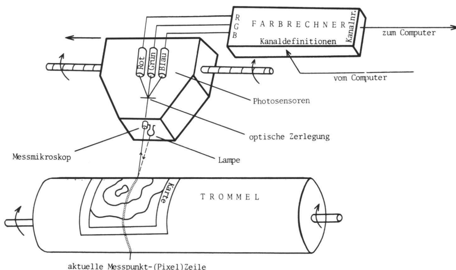
Abb. 3 Prinzipischema eines Mehrfarben-Scanners (aus [5]).
