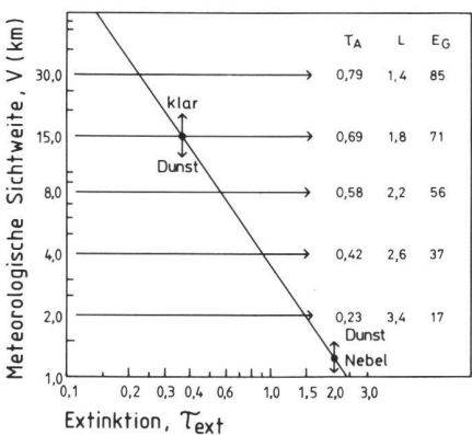
Abb.1 Meteorologische Sichtweite in Kilometer als Funktion der Extinktion \tau_{ext} bei \lambda=650 nm (nach Elterman [8]). Tabulierte Werte für vertikalen atmosphärischen Durchsichtigkeitsgrad \tau_A , atmosphärische spezifische Lichtausstrahlung L in Wsr^{-1}m^{-2} und Bestrahlungsstärke des horizontalen Bodens E_0 in Wm^{-2} berechnet wie im Text beschrieben für 40° Zenitwinkel der Sonne, Wellenlängenbereich 600 bis 700 nm und mittlere Hintergrundremission von 0,08. Im Falle fehlender Atmosphäre gilt eine meteorologische Sichtweite Unendlich, \tau_A=1 , L=0 und E_0=115 Wm^{-2} .
