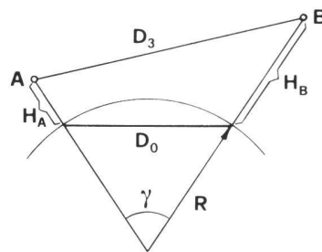
Abb. 7 Direkte Reduktion
