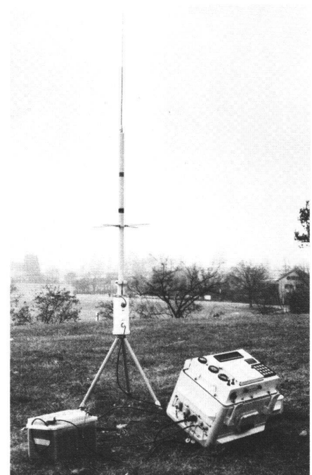
Abb.15 Dopplerempfänger Magnavox MX 1502 des Instituts für Geodäsie und Photogrammetrie der ETH Zürich in messbereiter Aufstellung (12-V-Batterie, Antenne, Empfänger/Mikroprozessor).
