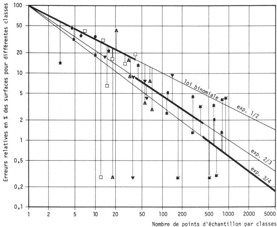
Fig. 9 Comparaison de l'erreur d'un échantillonnage estimée selon les lois de la statistique avec les résultats d'expériences pratiques dans 7 communes différentes (■ bâtim., ▲ routes, ▲ forêts, etc.).
