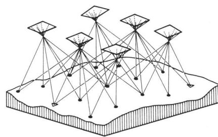
Fig. 2 Les relations géométriques entre 2 photos peuvent s'étendre à un grand nombre de photographies aériennes, ce qui permet de franchir de grandes surfaces avec un nombre minimal de points d'ajustage; procédé connu de triangulation aérienne.
