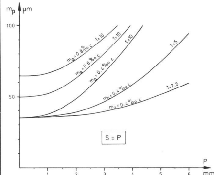
Abb. 1 Mittlerer Fehler m_p des Orthophotos in Abhängigkeit des Profilabstandes P, der Schlitzlänge S ( S = P ), der Geländecharakteristik T und des Profilierfehlers m_a , wobei sich m_p , c, P, S, T und m_a auf das bei der Datenerfassung verwendete Bild beziehen.
