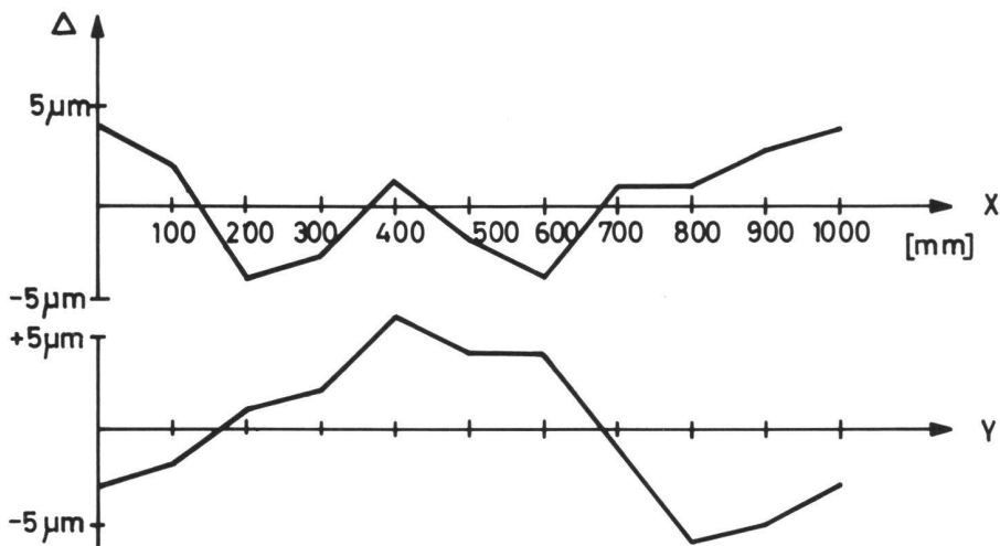
Abb. 5 Geradheit der X- und Y-Führungen am TA Nr. 4715. Die mittels eines genauen Stahlhlineales festgestellten Fehler sind kleiner als 5\text{ }\mu\text{m} .
