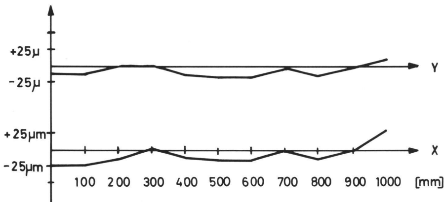
Abb. 6 Absolute Fehler im Massstab der Achsen X und Y des TA Nr. 4715. Die mittels eines Glasmassstabes festgestellten Fehler sind kleiner als 25\text{ }\mu\text{m} .
