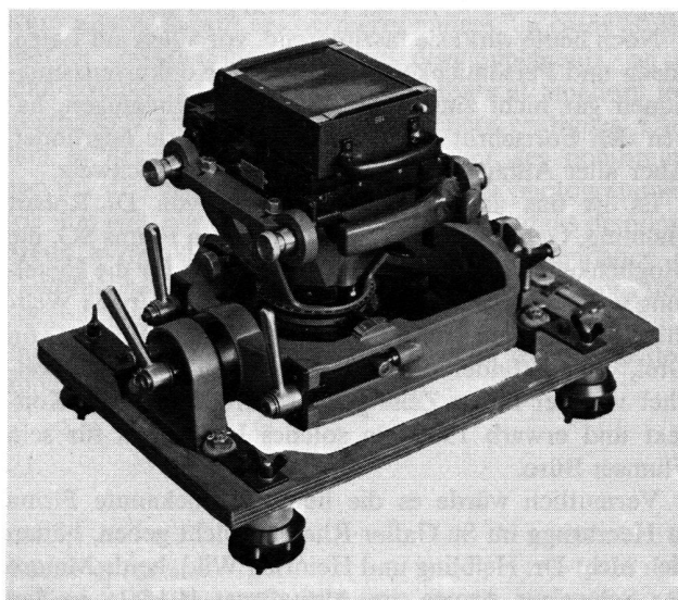
Abb. 3 Fliegerkammer C2 mit aufgesetztem Plattenmagazin
