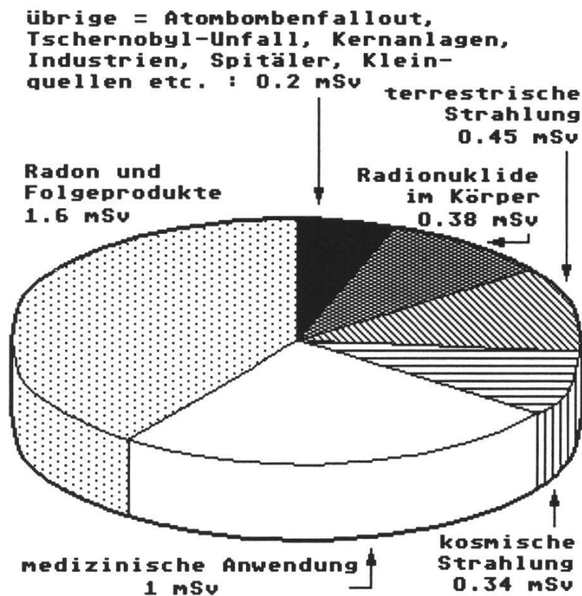
Abb. 4: Mittlere Strahlendosen der Schweizer Bevölkerung 1994. Summe der einzelnen Beiträge: 4 milli-Sievert (aus BAG-Jahresbericht 1994).
