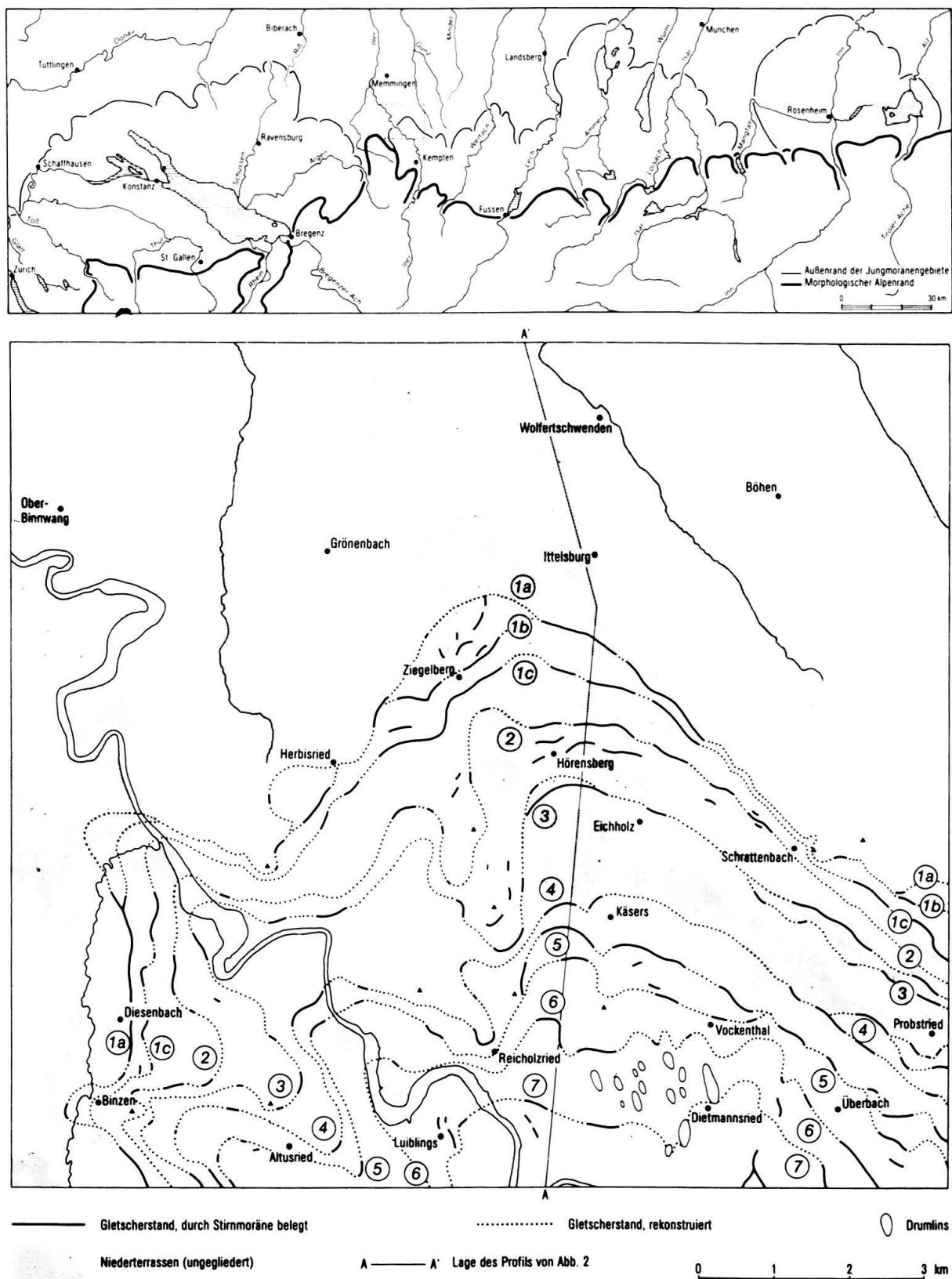
Fig. 1. Die Gletscherstände des würmzeitlichen Iller-Gletschers auf Blatt 8127 Grönenbach 1:25.000 und die Lage des Blattes im deutschen Alpenvorland. Aus Habbe 1985 (Reproduktion mit Bewilligung von Quartär).
