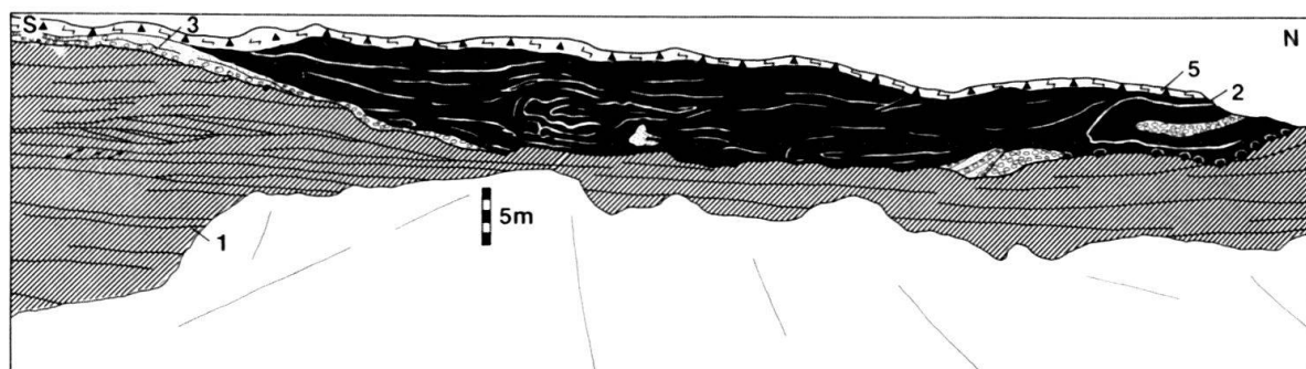
Fig. 7. Attisholzswald, chenal infraglaciale dont les sédiments sont fortement replissés. Légende des lithologies, voir tableau 1. Explication des numéros dans le texte.
