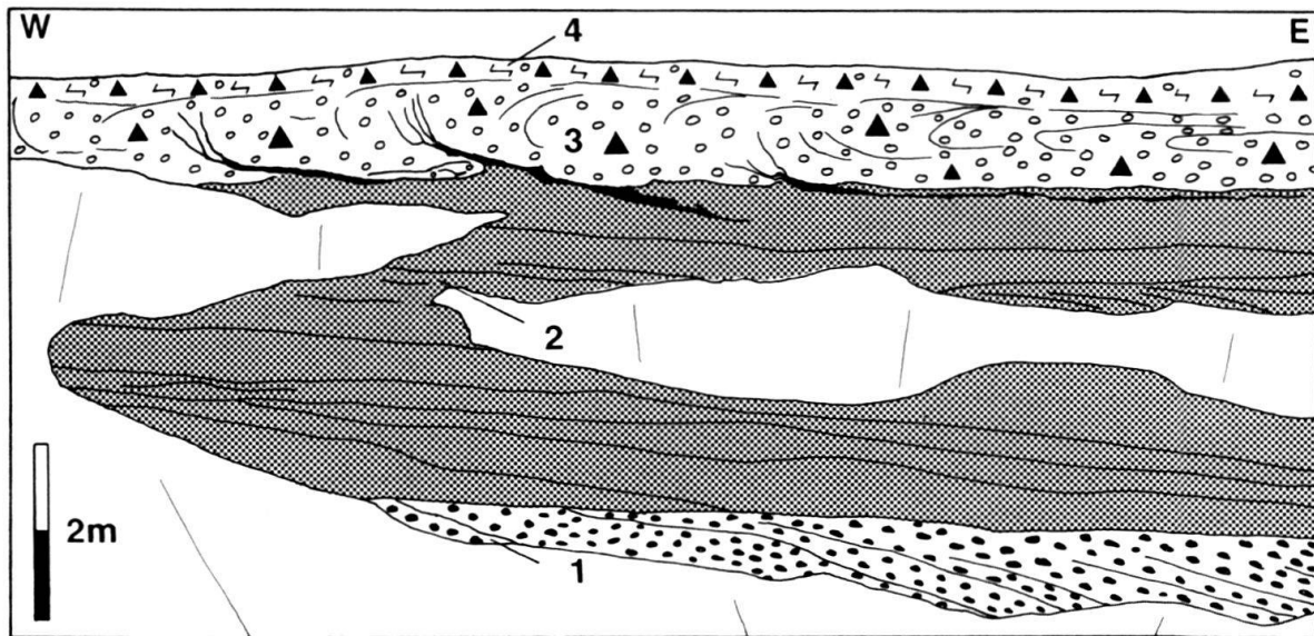
Fig. 10. Müntschemier, graviers fluviatiles basculés et revouverts par une diamictite (lodgement). Des filons sédimentaires pénètrent les graviers fluviatiles depuis la diamictite. Légende des lithologies, voir tableau 1. Explication des numéros dans le texte.
