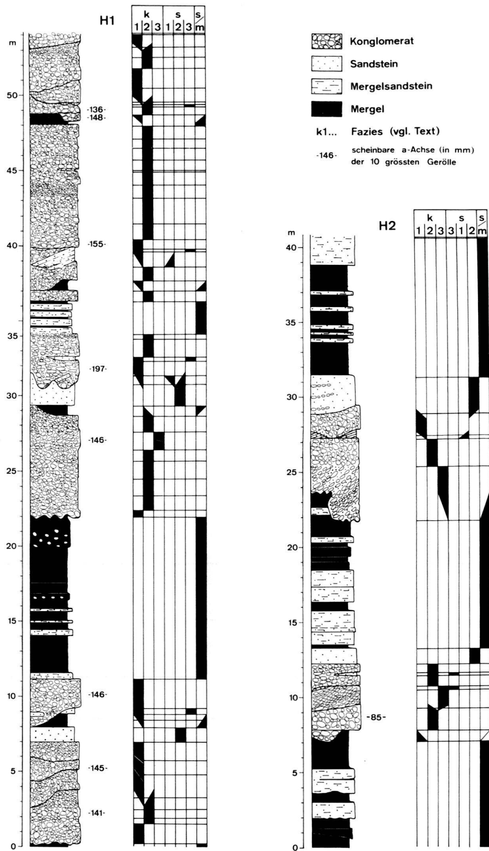
Fig.2. Profile durch die Konglomerat-Assoziation H1 und die Konglomerat/Mergel-Assoziation H2 . Lokaltäten: H1 = Hulttegg SG, Südseite, Strassenprofil zwischen Koten 818 und 872; H2 = Risitobel nördlich Stäfa ZH (697.650/233.950).
