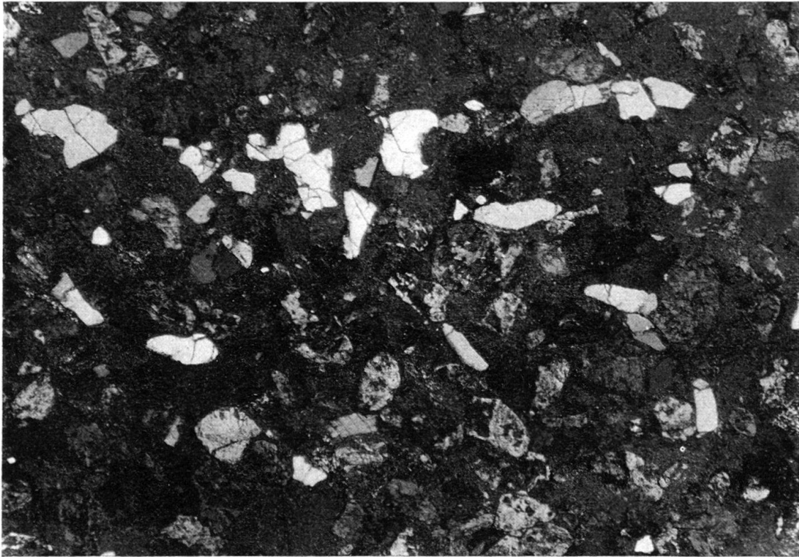
Fig. 2. Kristalltuff 227 aus der «Grenzbitumenzone» des Monte San Giorgio (Schnitt \parallel s; 24fache Vergr.; + Nicols). Quarz (weiss) mit Korrosionsumrissen und Sanidin-Typ A (grau, stark zersetzt).
