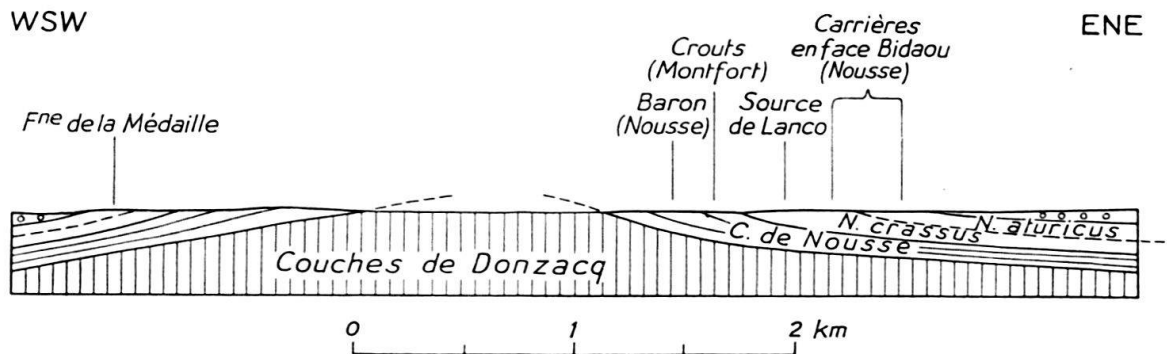
Fig. 2. Schematisches Profil durch die Antiklinale von Montfort, umgezeichnet nach BURGER, CUVILLIER & SCHOEFLER (1945, Fig. 2).
