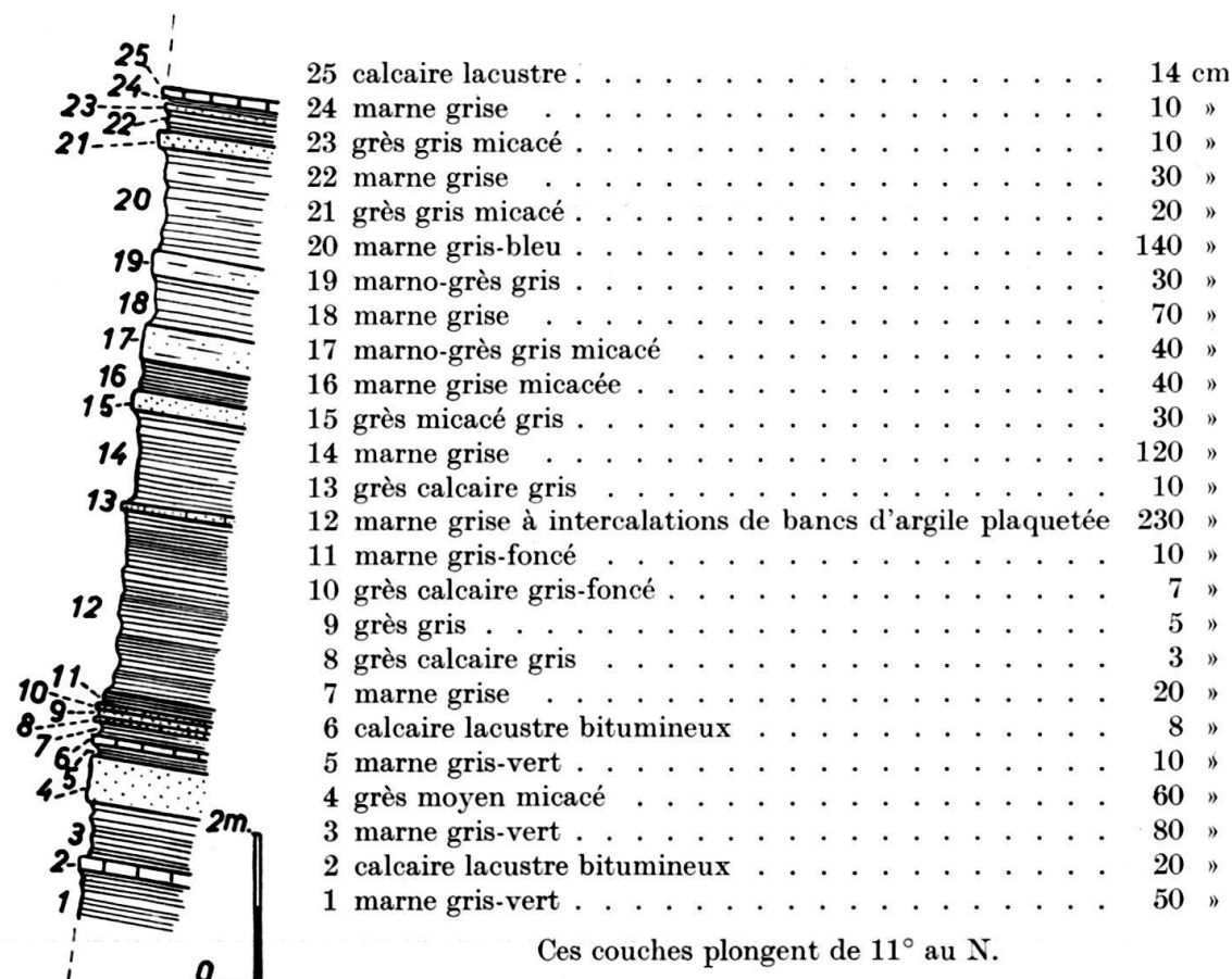
Fig. 17. Coupe stratigraphique des Ligrines (ravin de la Morges).
