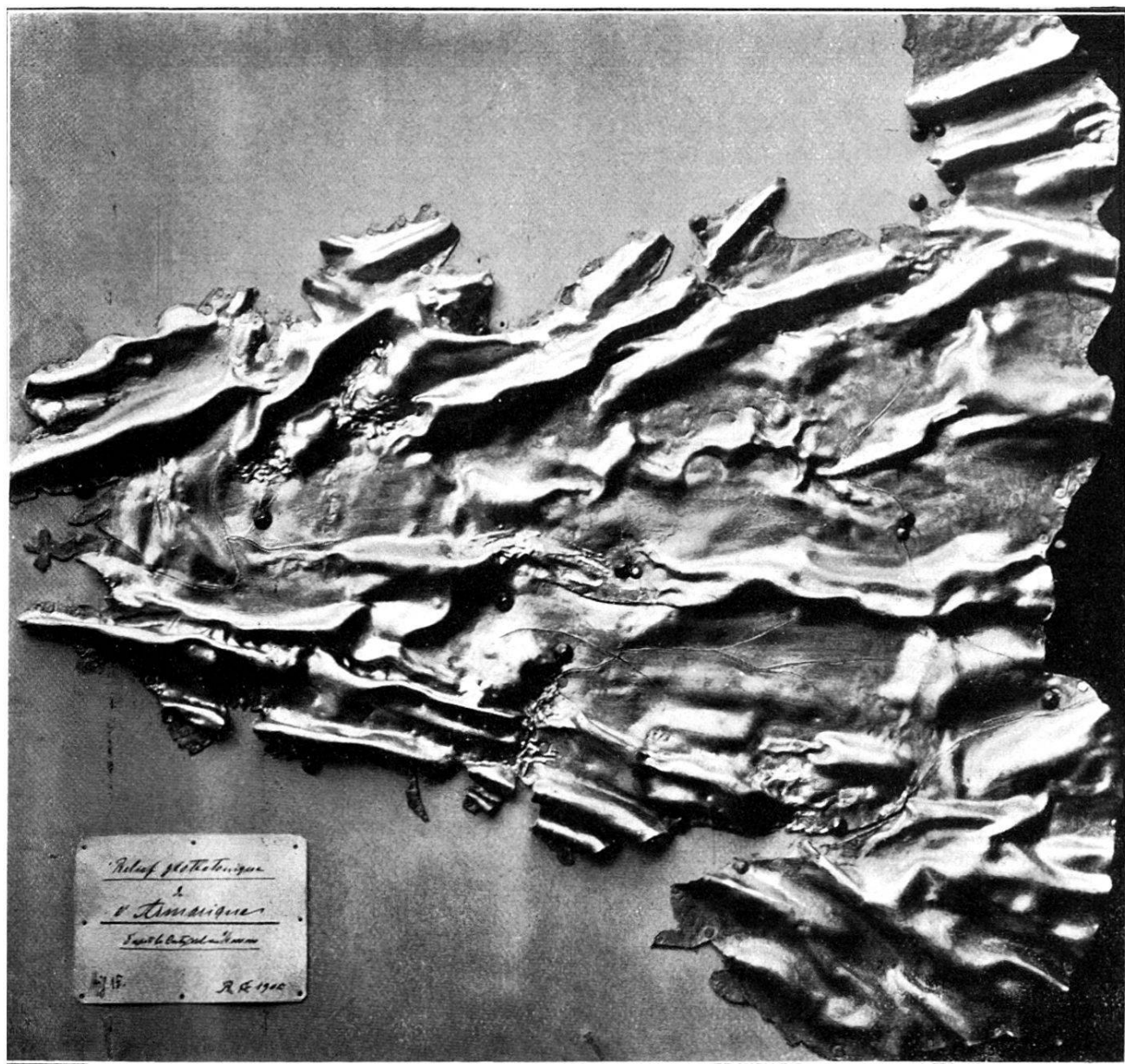
FIG. 3. — Le Horst armoricain.
