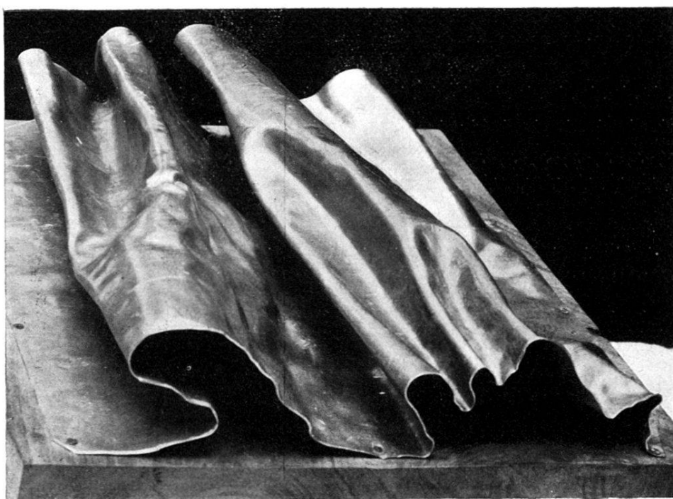
FIG. 2. — Plis couchés ramifiés.
