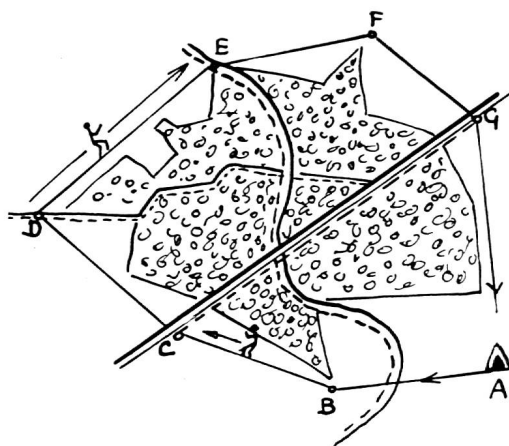
AA' : erreur de fermeture
