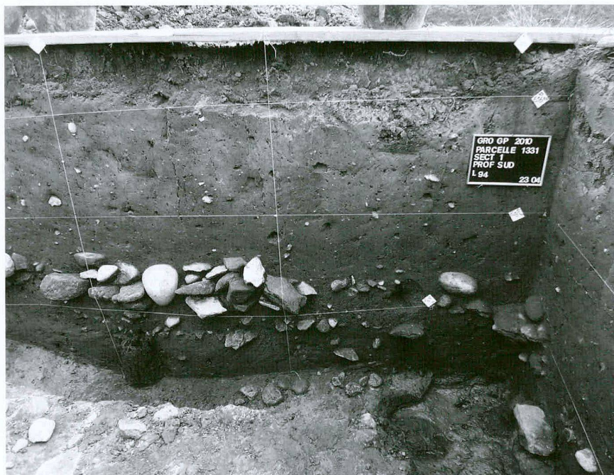
Fig. 13 Grolley/Au Gros Praz. Vue en coupe des deux empièvements successifs et de l'un des poteaux stabilisant le terrain en bordure de la dépression humide
