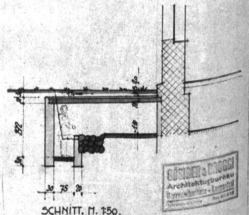
SCHNITT, M. 1:50. MASSAUFNAHME VOM 14. APRIL 1945. BÖSIGER UND BROGGI, ARCH. BÜRO.
