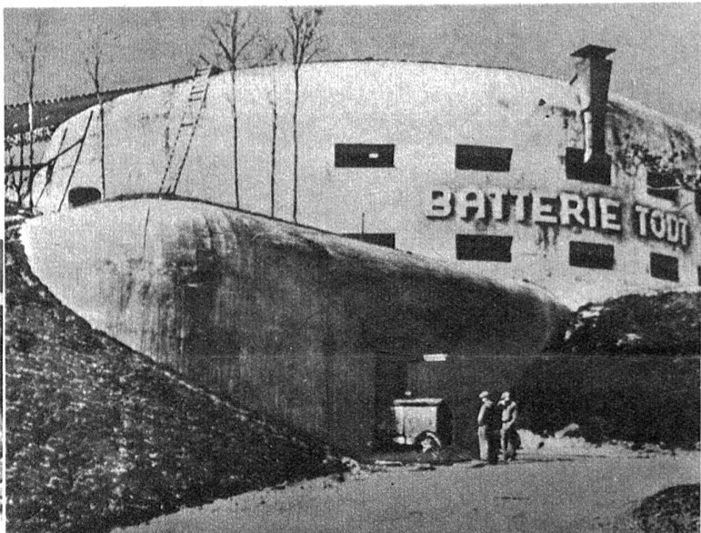
Das Oberkommando der deutschen Wehrmacht teilt mit, dass der Befestigungswall, der von der französisch-spanischen Grenze bis zum Nordkap reicht, fertig gestellt ist. Unser Bild zeigt einen massiven Betonbunker einer Fernkampfbatterie an der Atlantikküste
