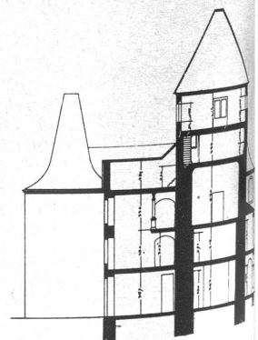
Querschnitt. Durch seine Mauerstärke (zwei Meter) ist der alte Wehrturm als ältester Bauteil deutlich erkennbar
