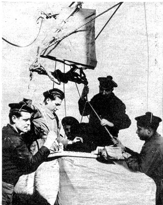
Der Beobachter legt in der Gondel seine Bordinstrumente und den Fallschirm zurecht.
