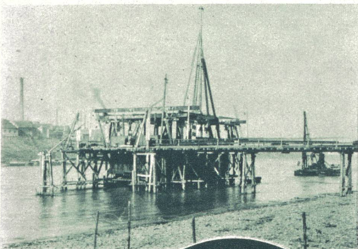
Beginn der Bauarbeiten an der Basler Dreirosenbrücke , die einige hundert Meter oberhalb der Grenze die beiden Ufer verbinden soll. Die Versenkung der ersten Caissons. Phot. Gallas, Zürich.
