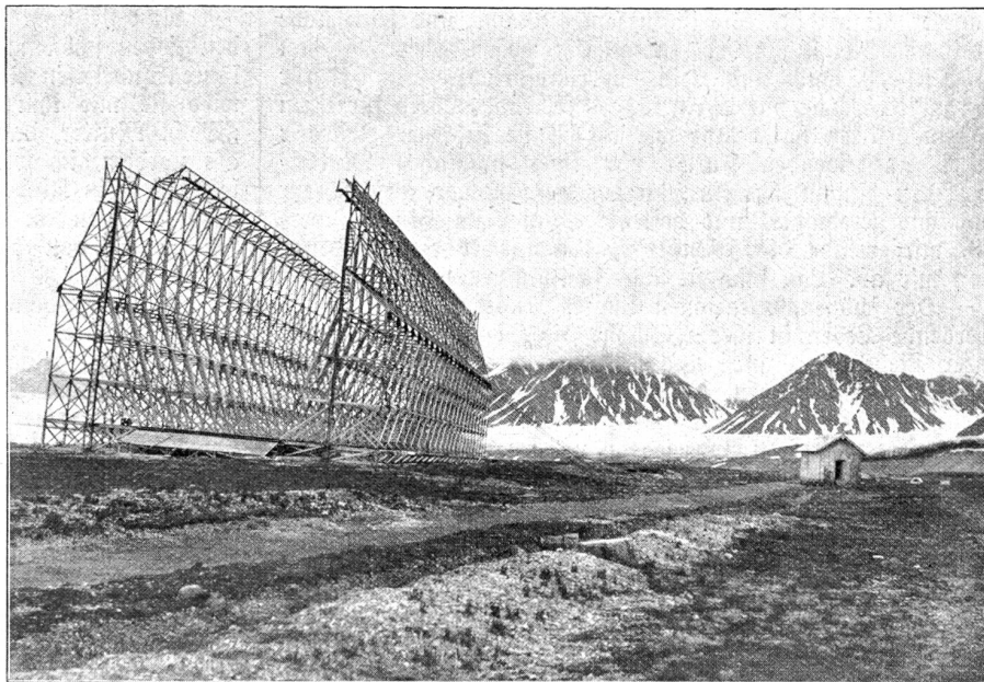
Luftschiffhalle in der Königsbucht auf Spitzbergen. Wurde von Amundsen und dann von Robile für die Nordpolexpeditionen benutzt, von welchen letztere in bekannt tragischer Weise endete.
