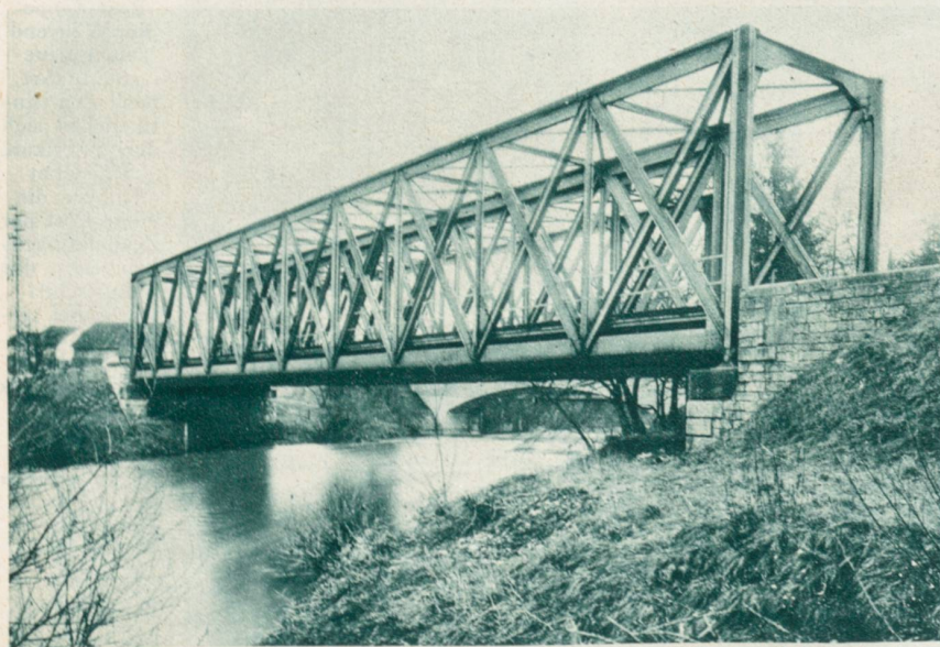
Vor 40 Jahren, am 14. Juni 1891, stürzte der Zug der Jura-Simplon-Bahn mitsamt der Brücke bei Münchenstein (Baselland) in die Birs. Das Unglück forderte 73 Tote. Verletzt wurden an die 200 Personen. Unser Bild zeigt die nachher neu-erstellte Brücke.
