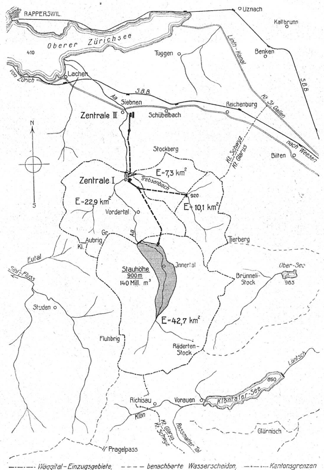
Das Wäggitälwerk. Kliffsee „Schweiz. Bauztg.“ Die Einzugsgebiete des Kraftwerks Wäggitäl. — 1:200,000.
