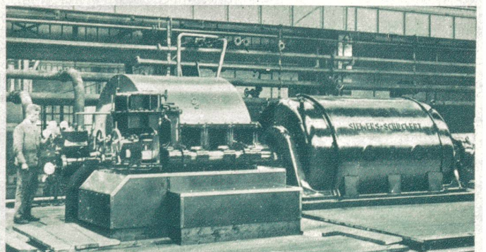
Die grösste Radialturbine der Welt ging kürzlich aus dem Mühl- heimer Werk der Siemens-Schuckertwerke hervor. (Phot. Keystone)
