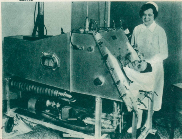
Bett in einen luftdichten Behälter gelegt, wobei nur der Kopf herausragt. Eine elek- trische Pumpe zieht dann die Luft aus dem Behälter, ungefähr 15mal jede Minute, und da jedesmal der Luftdruck in dieser Weise vermindert wird, müssen die Lungen des Kranken sich ausdehnen, ob er will oder nicht. Phot. Keystone.
