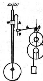
Schema (links) und Ansicht (rechts) einer Pendeluhr, nach der Erfindung konstruiert.
