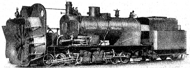
Schneeschaufler der Berninabahn. — Reiner Adhäsionsantrieb. Der Antrieb des Schlagrades erfolgt durch separate Zweizylindermaschine
