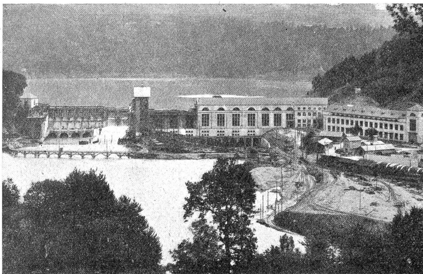
Das Hare-Stauwerk bei Mühleberg im Baustadium Ende August. Staudamm — automat. Schleusen — Maschinenhaus, unvollendet, Schalt- und Transformatorenhaus.
