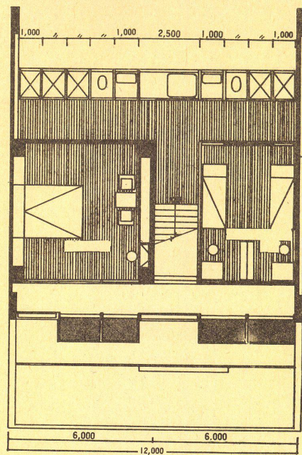
19 Grundriß Eingangsgeschoß 1:200.
