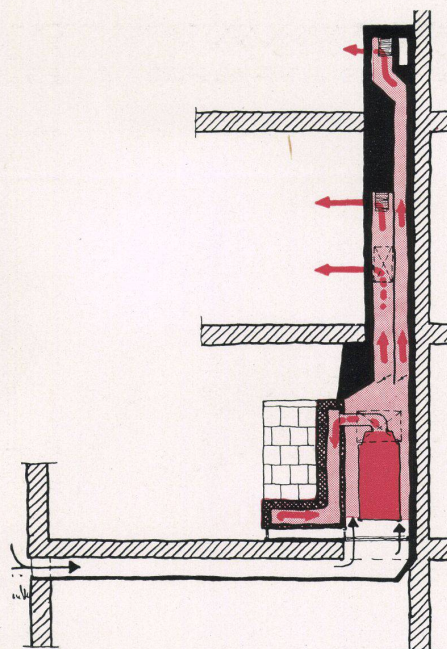
Warmluftsammlerheizung in Kombination mit Kachelofen. Schematischer Schnitt. Im Sommer zur Frischluftzirkulation verwendbar.
