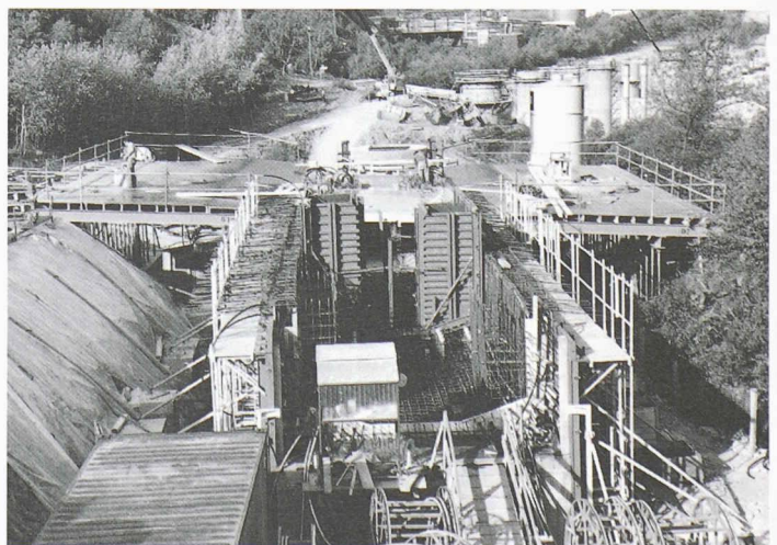
Fig. 3.- Aire de fabrication avec moules de coffrage
