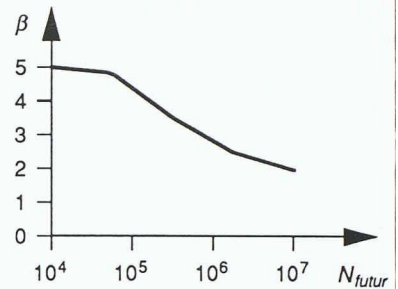
Fig. 5. — Relation schématisée entre indice de fiabilité \beta et nombre de cycles de charge N_{\text{futur}} pouvant encore être appliqués
