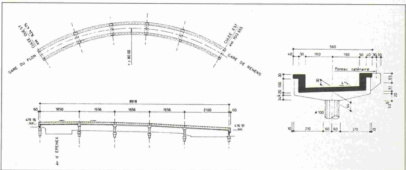
Fig. 24. - Pont d'Epenex: plan général.
