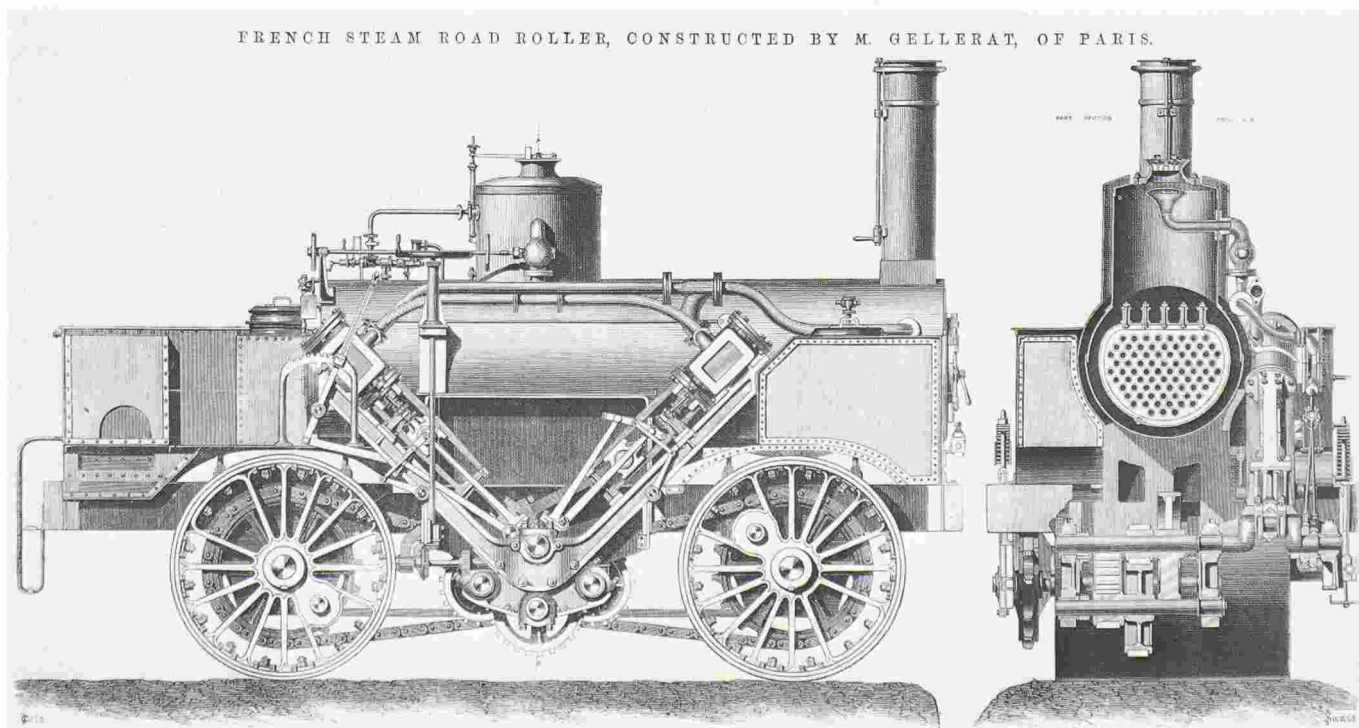
Fig. 4. – Rouleau à vapeur Gellerat, système Ballaison amélioré (1867), d'un poids de 22 à 29 tonnes, utilisé à Paris.
