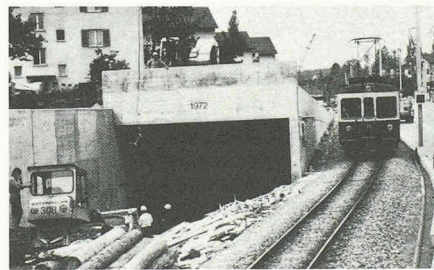
2121 Worblaufen bis Bern 1963-74 Unterirdische Führung der SZB-Bahn Worblaufen-Felsenau-Bern HB, Doppelp- spur für Taktfahrplan, Ing. Bernet + Wey- neth
