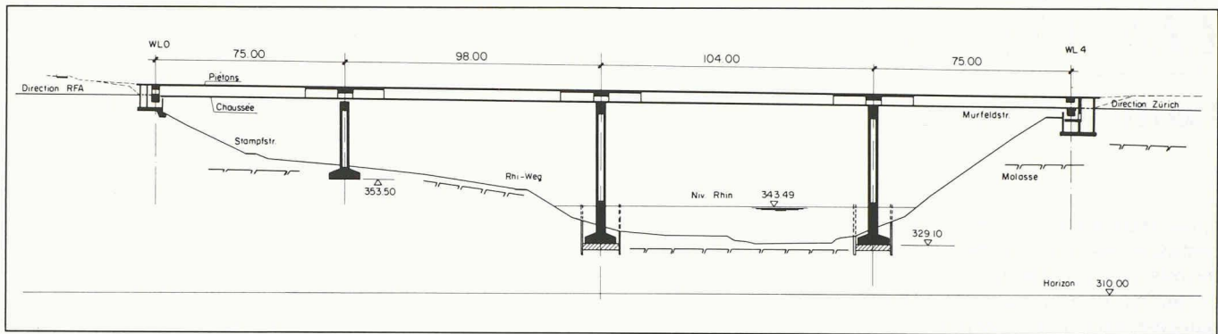
Fig. 2. — Coupe longitudinale.
