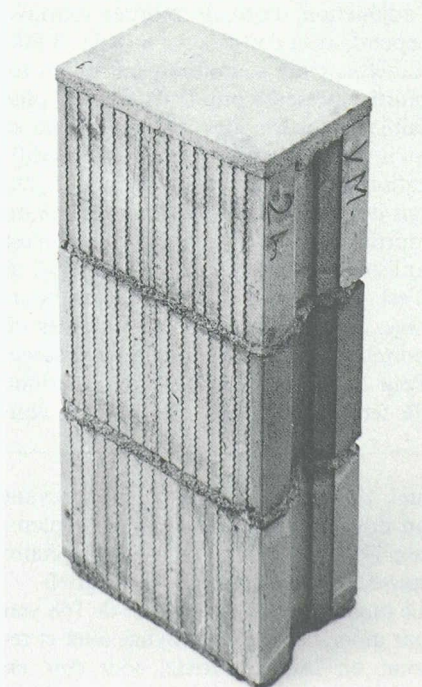
Fig. 2. — Muret de 3 briques avec couche de mortier d'égalisation sur les surfaces d'appui.
