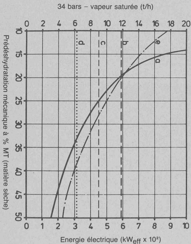
Exemple des données d'exploitation d'une station d'incinération des boues d'épuration des eaux usées pour 360 000 de population équivalente:
