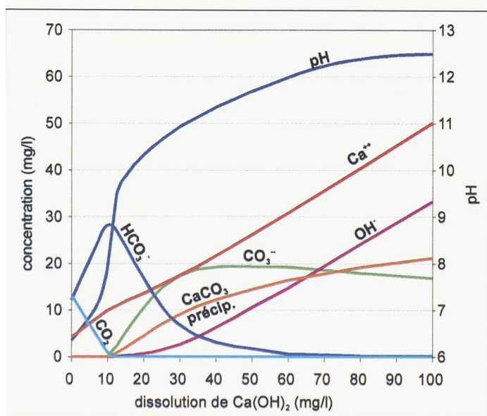
Fig. 3. - Modèle de dissolution de la portlandite dans une solution aqueuse au chimisme du lac du Naret (pH = 6,4; Ca²⁺ = 4 mg/l; HCO₃⁻ = 12 mg/l).
