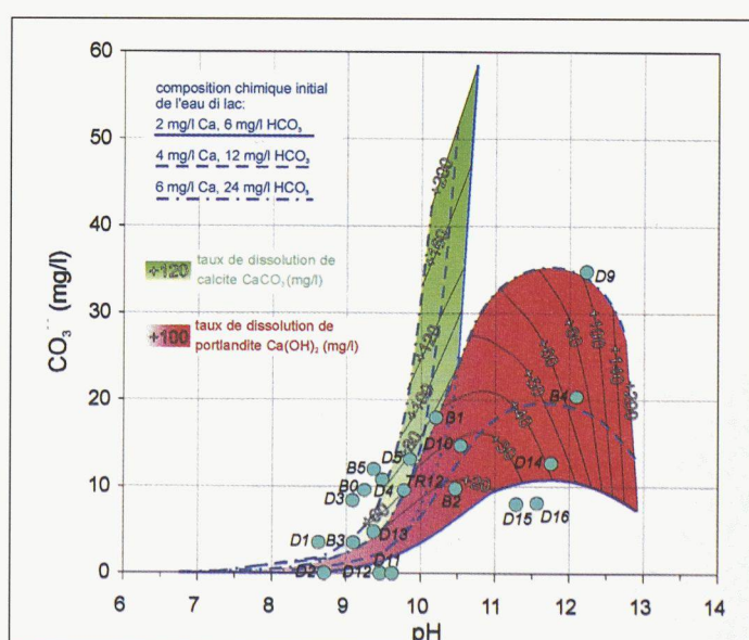
Fig. 5. - Diagramme pH-CO₃²⁻ avec les domaines de dissolution de portlandite (en rouge) et de calcite (en vert) par rapport au chimisme de l'eau du lac, avec pH et concentration en CO₃²⁻ des eaux sortant des drains. Les drains dans le domaine de la portlandite témoignent d'une dissolution de l'écran d'étanchéité.
